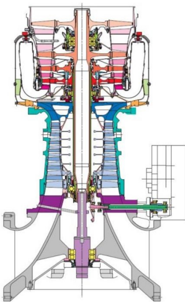
ASE40V 横剖图
