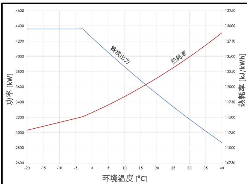
额定功率vs 环境温度
